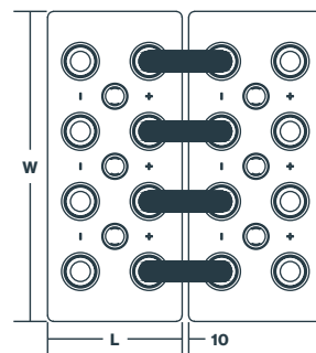
18 OPzS-ET 2250 to 26 OPzS-ET 3250
